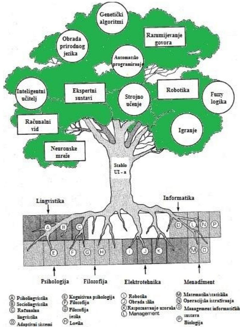
Slika 1: Stablo UI-e
