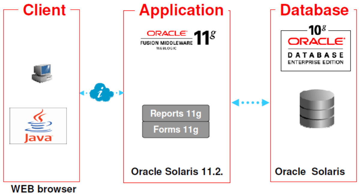
Slika 16: Infrastruktura - softver
