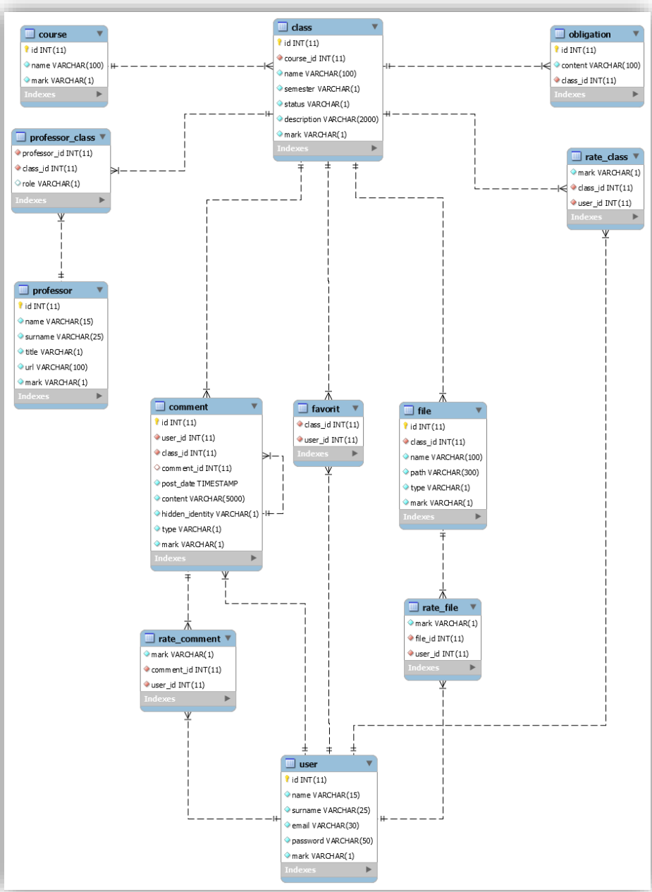
Slika 22. ERD Model
