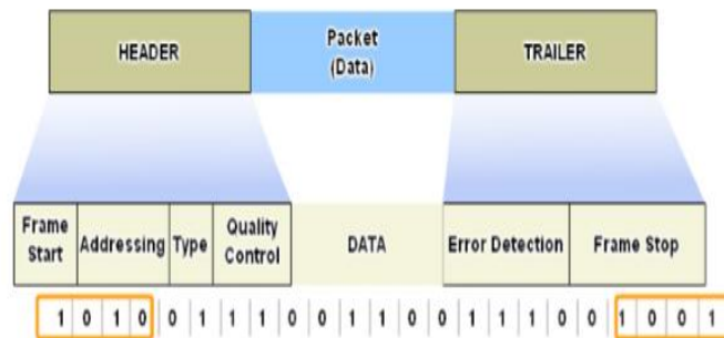
Slika 8. Opći oblik frame-a odnosno okvira(M.Korač;D.Car:Uvod u računalne mreže:2014:32)
