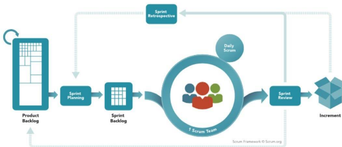
Slika 9. SCRUM
