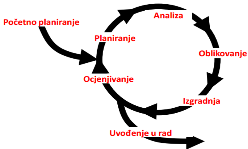
Slika 6: Iterativni pristup
