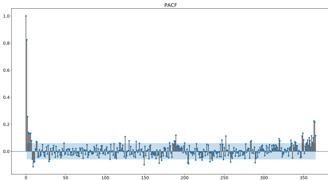
Slika 7.2: PACF prikaz
