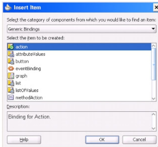
Slika 18 – dodjeljivanje akcije
