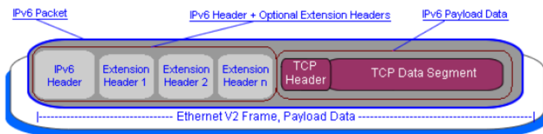
Slika 10. IPv6 enkapsulacija.
