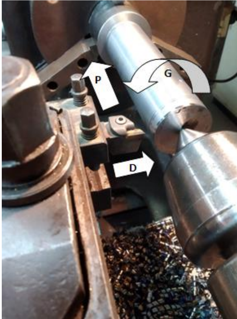
Slika 8. Prikaz gibanja na tokarskom stoju
