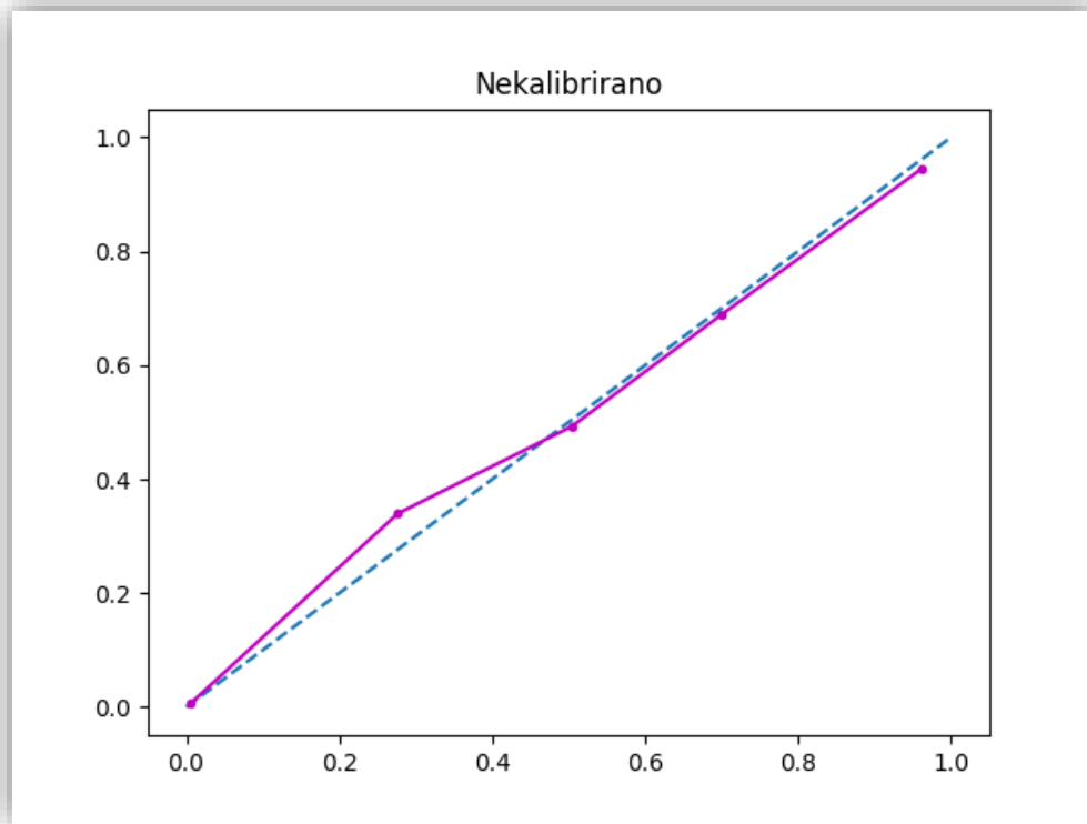
Slika 42. Krivulja kalibracije
