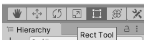
Slika 7 - Rect tool
