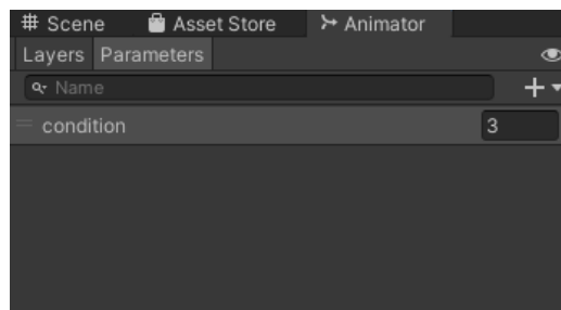
Slika 33 - Animator parametri
