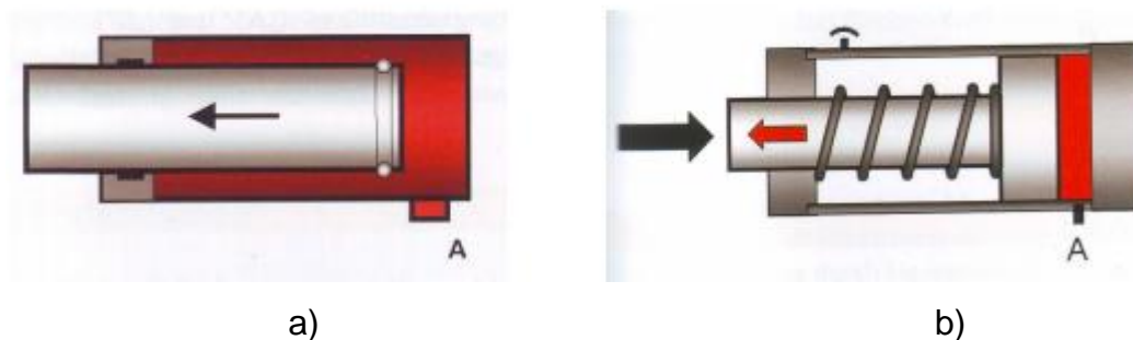
Slika 12 Jednoradni cilindar
