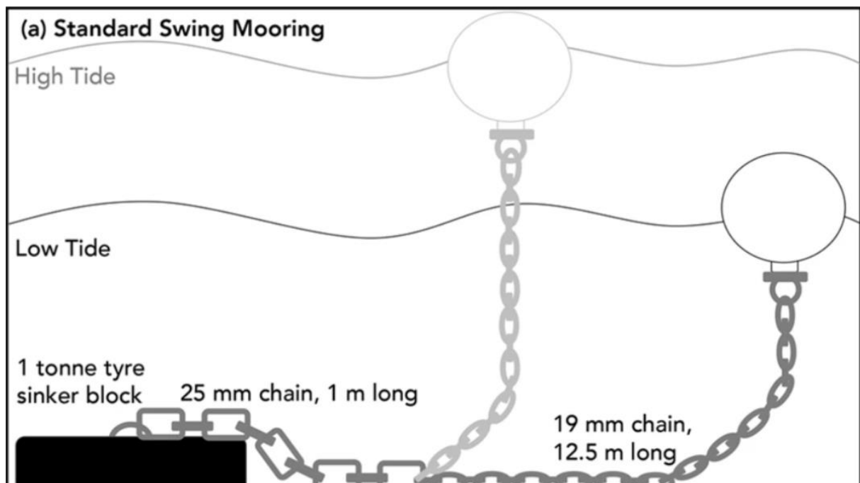
Slika 27: Prikaz tradicionalnog veza čiji se lanci nalaze na dnu.
