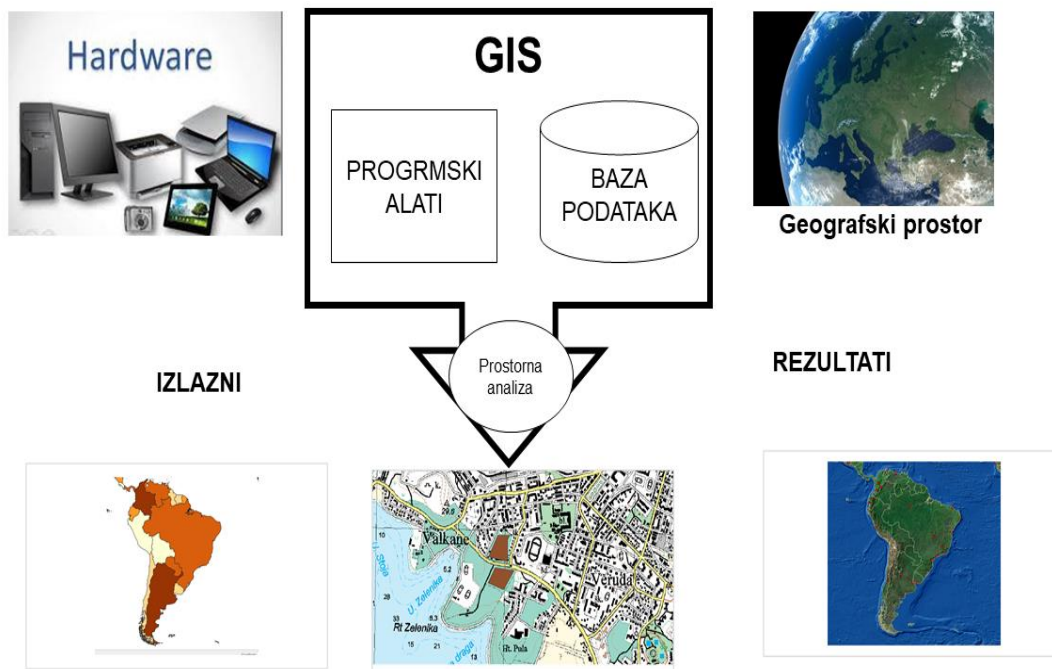
Slika 1. Proces GIS-a
