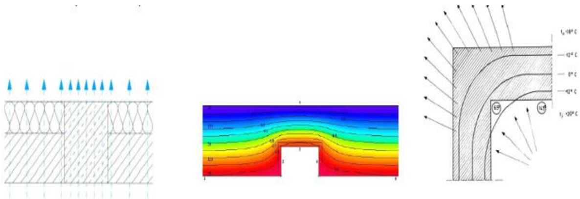
Slika 9. Toplinski mostovi
