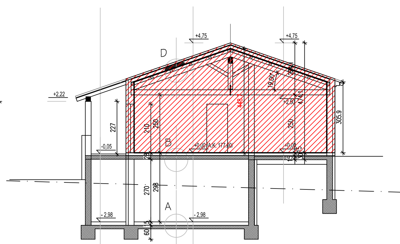
PRESJEK A-A MJ 1:100
