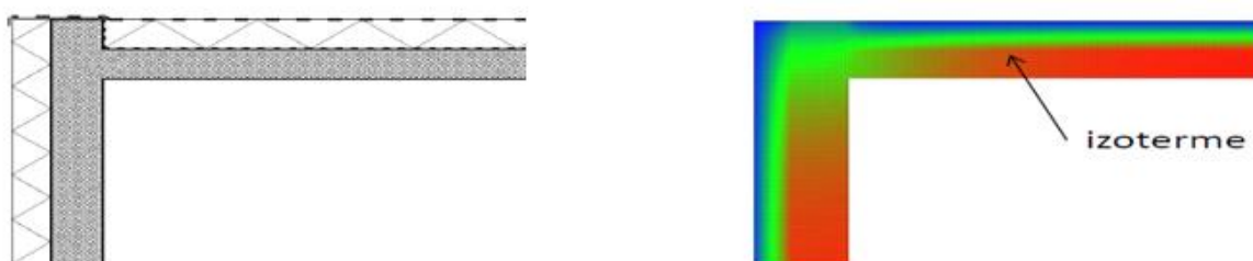
Slika 11. Toplinski most I – presjek konstrukcije
