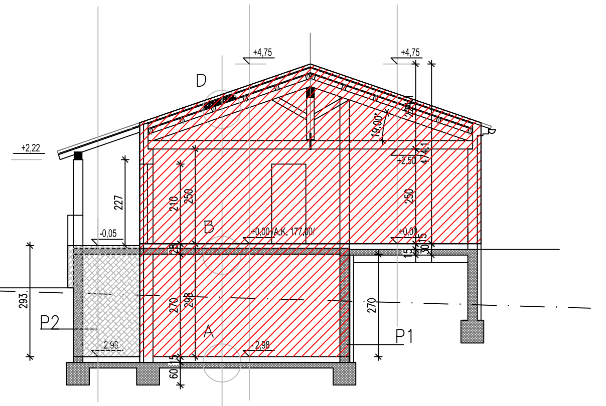
PRESJEK A-A MJ 1:100
