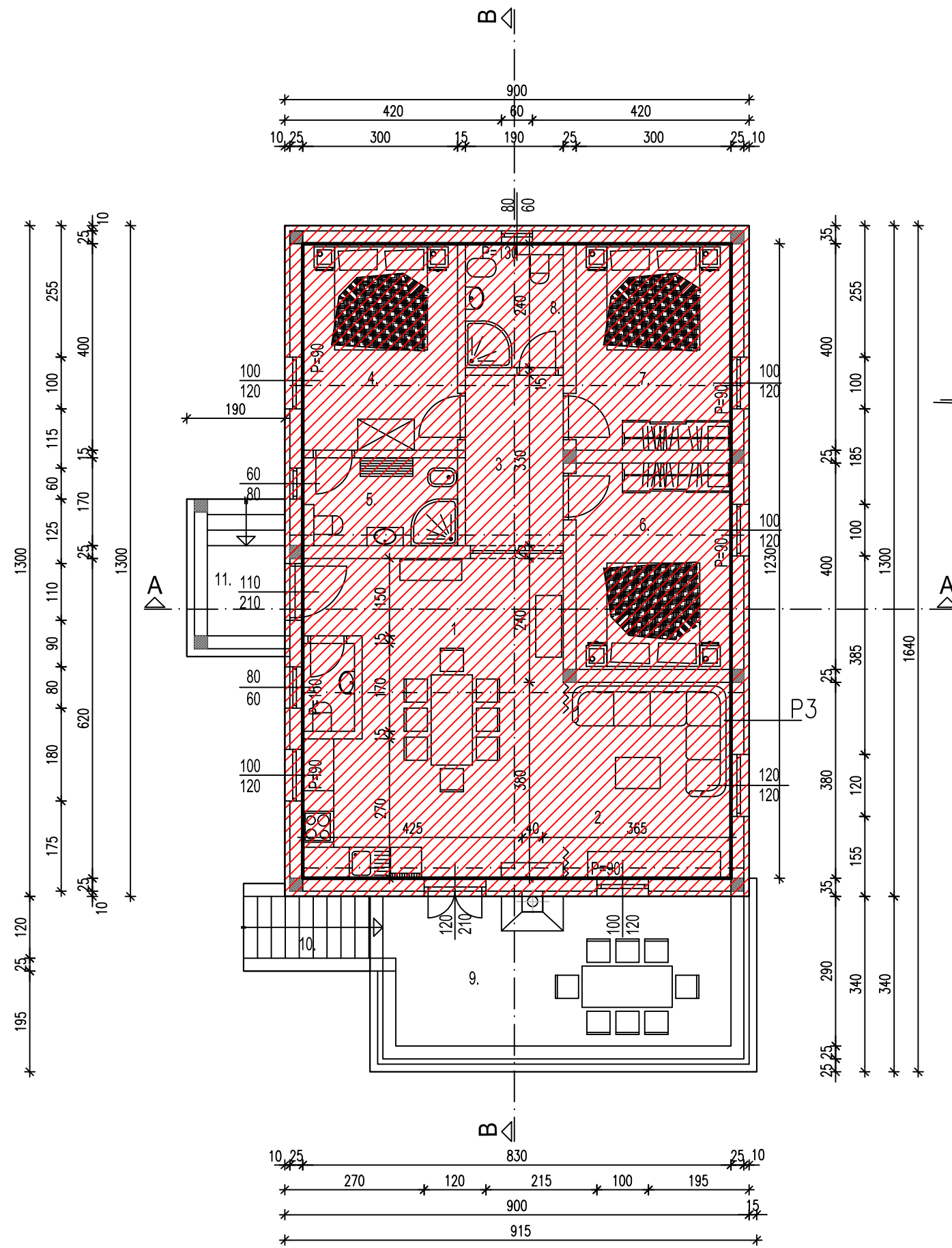
TLOCRT PRIZEMLJA MJ 1:100 ISKAZ VOLUMENA I OBRAČUNSKIH VELIČINA
