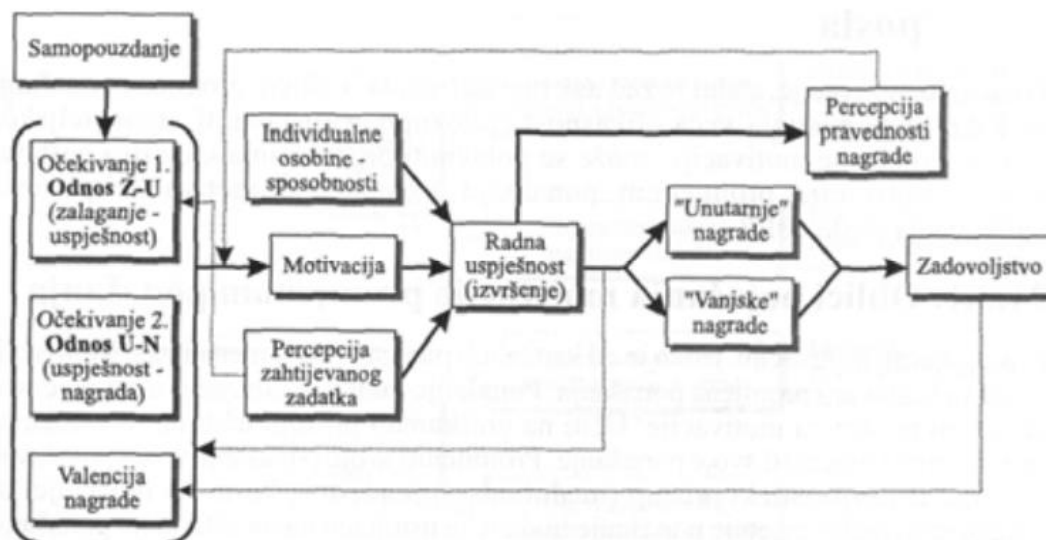
Slika 4. Porter-Lawlerov model očekivanja
