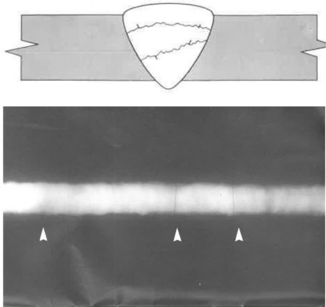
Slika 59. Primjer pukotina vidljivih radiografskim ispitivanjem (Izvor: https://www.nde-ed.org )
