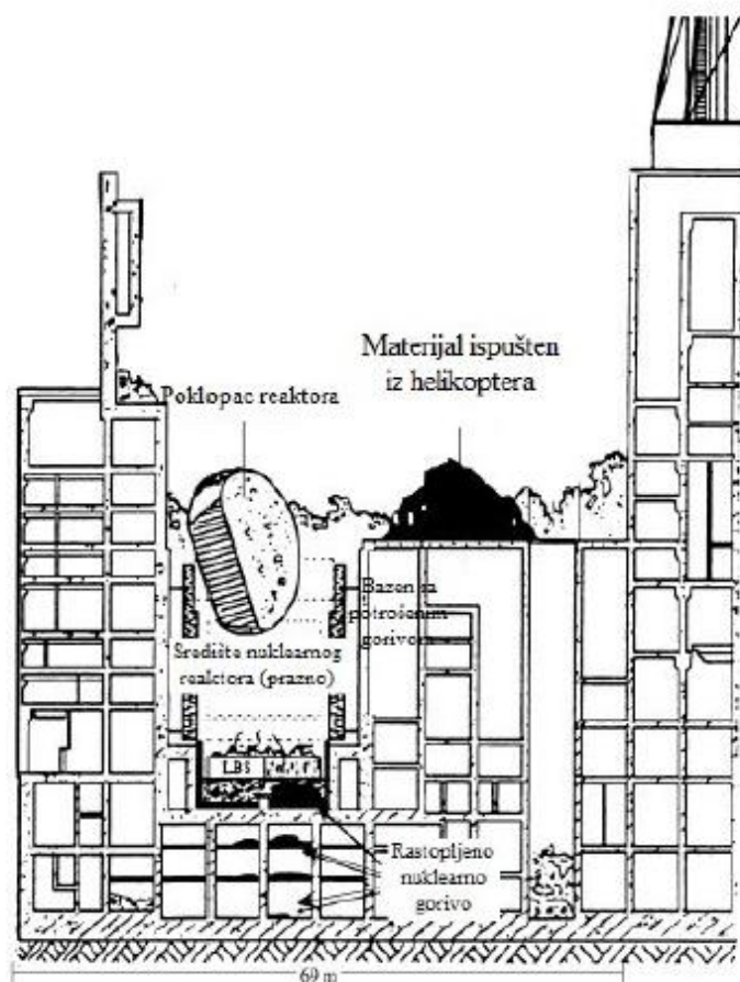
Skica 1: Presjek reaktora
