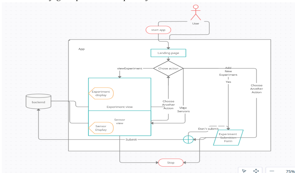
Slika1. UML dijagram prve inačice aplikacije
