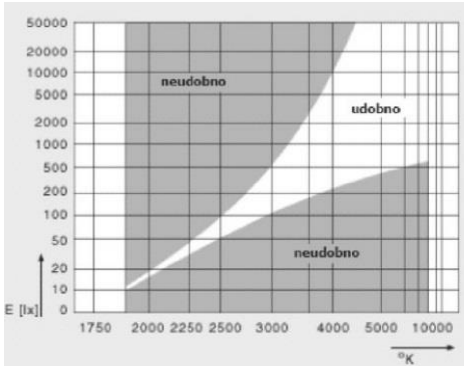
Slika 21. Kruithof-ov dijagram ( E[lx] -razina osvjetljenosti, ^{\circ}K -temperatura boje)
