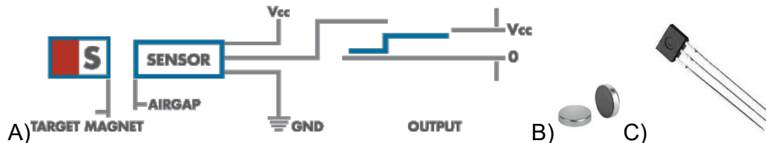
Slika 8. Mjerenje otvorenosti ljuštura dagnji pomoću Hall senzora magnetskog toka: A) princip rada Hall senzora; B) magneti; C) Hall senzor.
