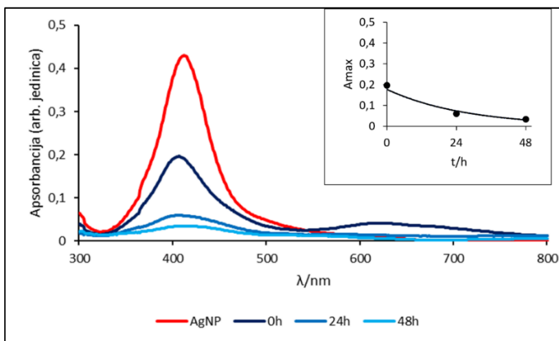
Slika 18. Promjena apsorpcijskog spektra i apsorpcijskog maksimuma alginata (1 \mu\text{g/mL} ) i AgNP-a (0.02 \mu\text{g/mL} ) snimanog u ASW kroz 48 h.
