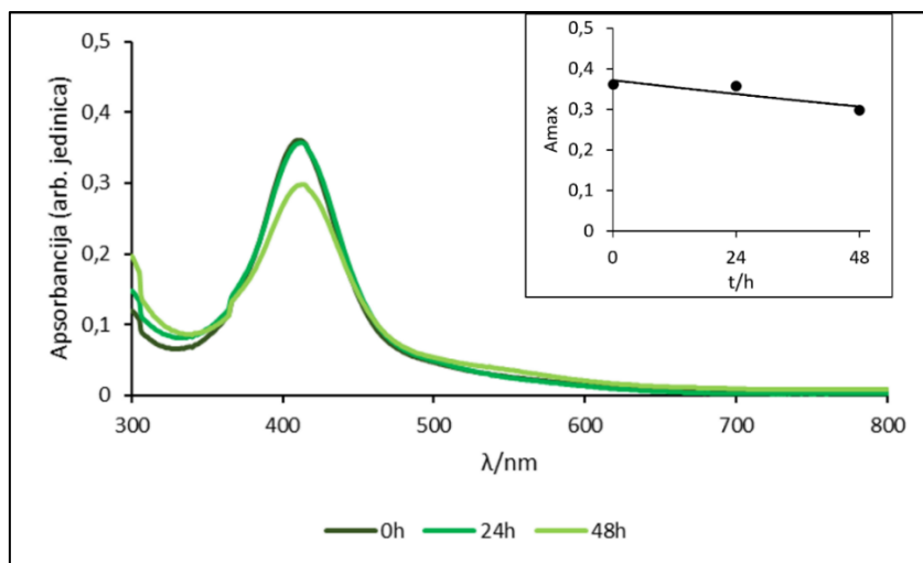
Slika 17. Promjena apsorpcijskog spektra i apsorpcijskog maksimuma alginata (1 \mu\text{g/mL} ) i AgNP-a (0.02 \mu\text{g/mL} ) snimanog u ultračistoj vodi kroz 48 h.
