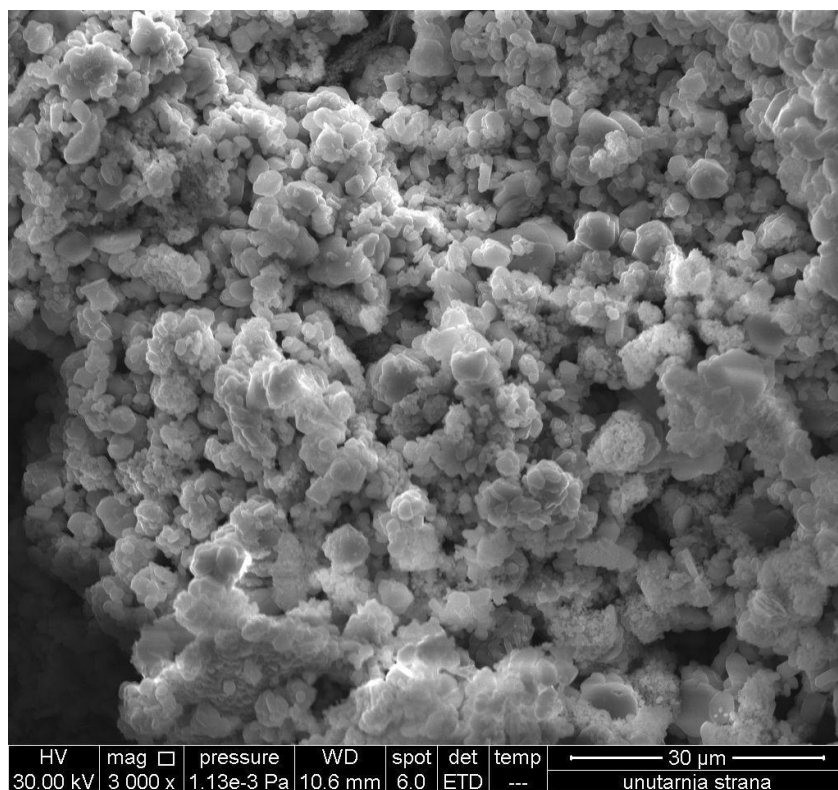
Slika 30: Unutarnja strana cijevi uvećana 3000X
