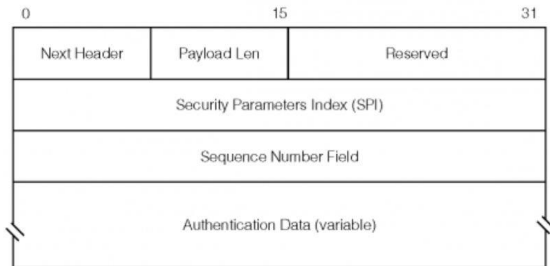
Slika 6. Authentication Header
