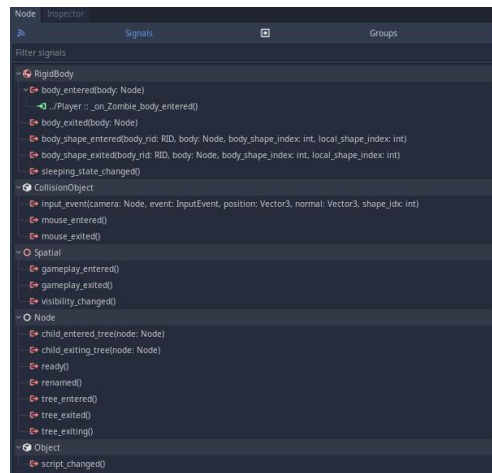
Slika 37: Primjer signala u Godot-u
