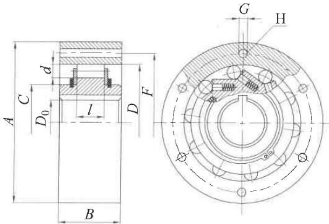
Slika 10. Valjni zadržać
