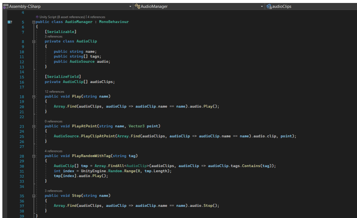
Slika 50 - Klasa AudioManager
