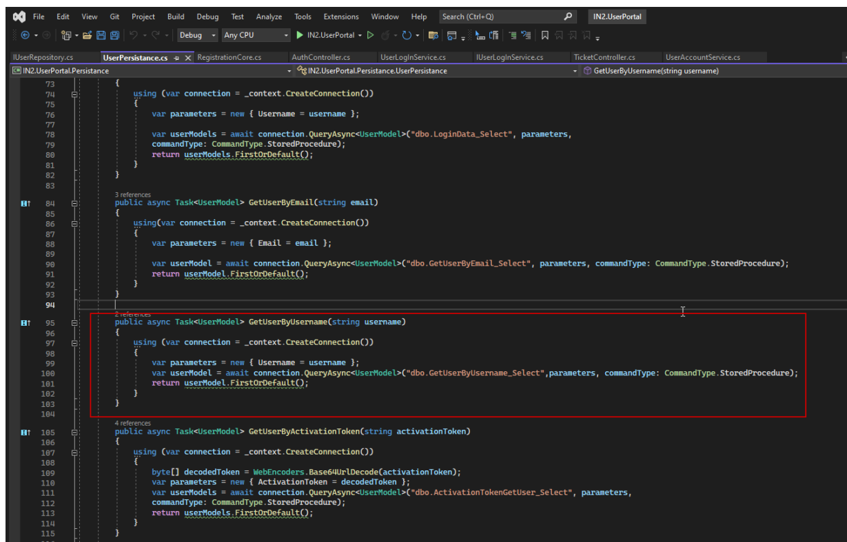
Slika 31. UserPersistence klasa
