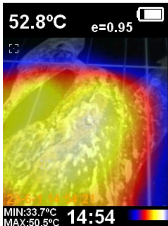
Slika 39. Prljavština na fotonaponskom panelu snimljena termalnom kamerom
