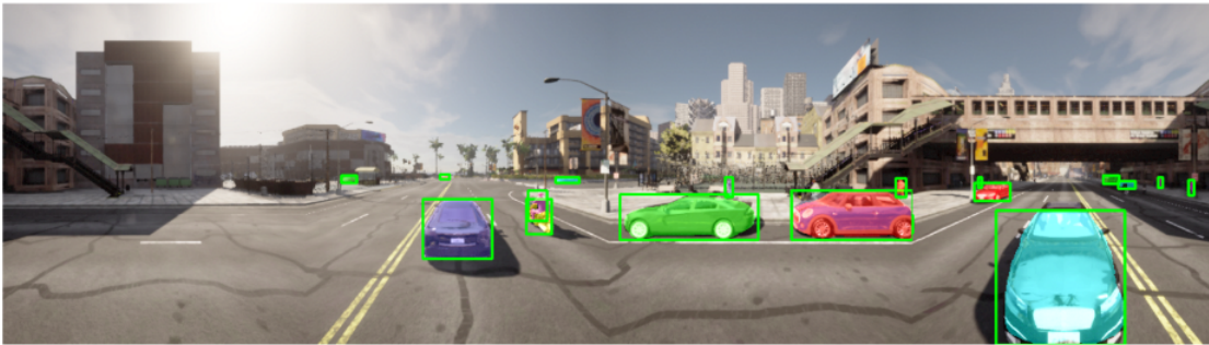
Mask R-CNN
