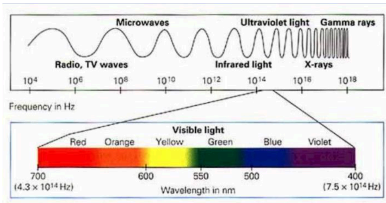
Slika 3.3.1. Elektromagnetski spektar [4]
