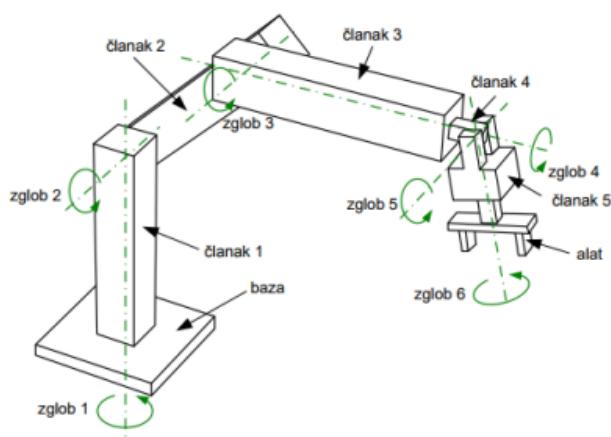
Slika 25 Robotski manipulator
