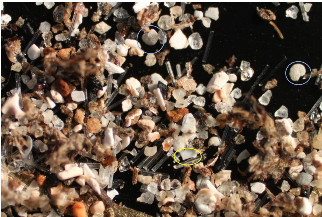
Slika 13. Postaja F1, jesensko uzorkovanje, dubina jezgre 26-28 cm, frakcija 0,125-0,25 mm, ●- foraminifere, ●- ostaci ljušturica. Napomena: duljina mjerila na Slici 12. primjenjiva je i na ovu sliku (autor: Andreja Kokorović).
