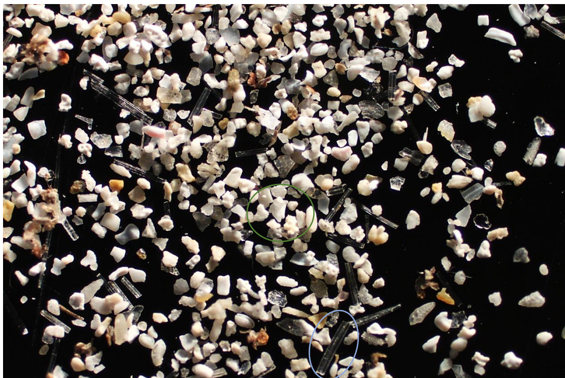
Slika 25. Postaja: područje rasta cvjetnice C. nodosa , ljetno uzorkovanje, dubina jezgre od 0-2 cm, frakcija 0,063-0,125 mm, ●- fragmenti ljuštura školjkaša i kućica gastropoda, ●- spikule spužvi. Napomena: duljina mjerila na Slici 18. primjenjiva je i na ovu sliku (autor: Andreja Kokorović).
