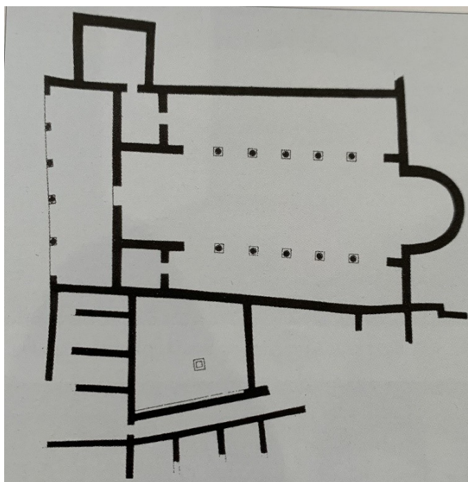
Slika 20. Tlocrt crkve i samostana (T. Marasović, 2011., 369.)
