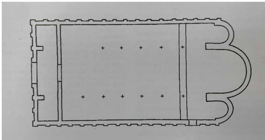
Slika 14. Tlocrt bazilike sv. Ivana Evanđelista, prema M. Jurkoviću (T. Marasović, 2009., 432.)
