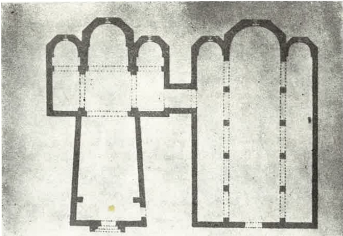
Slika 11. Tlocrt sv. Klementa (slika lijevo) i Sv. Mihovila (slika desno)
