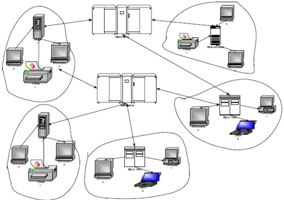
Slika 6: Hibridna arhitektura
