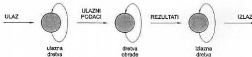
Slika 12. Cikličke dretve u ostvarenju cjevovodne obrade (Izvor: Budin L., Golub M., Jakobović D., Jelenković L. : Operacijski sustavi , 3. Izdanje, Zagreb, 2013(str69.))
