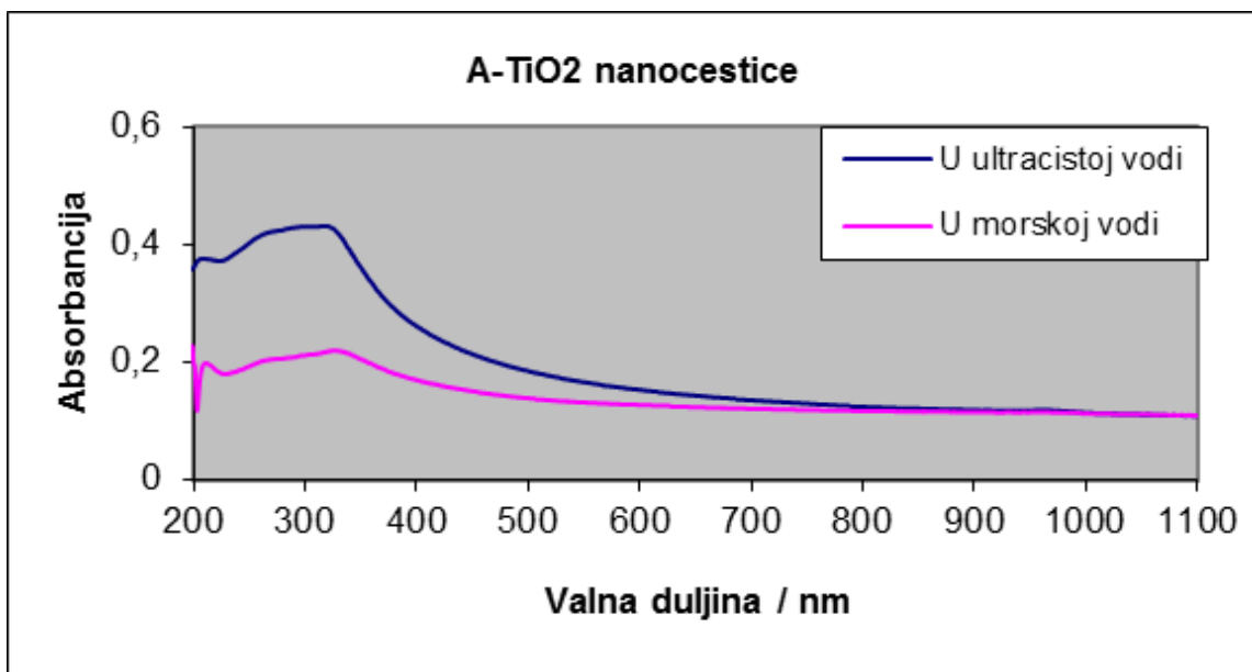
Graf 7. UV spektrofotometrijske krivulje A-TiO 2 NPs: plavom bojom prikazana je krivulja nanočestica anatsnog titanijeva(IV) oksida (100 μg/L) u ultračistoj vodi dok je ružicastom linijom prikazana krivulja istih čestica u umjetnoj morskoj vodi.
