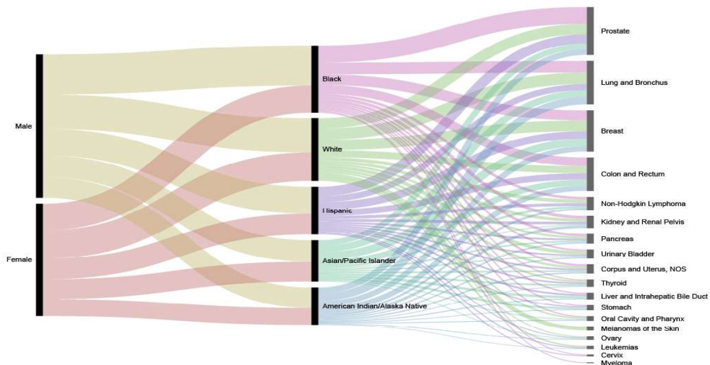
Slika 16. Prikaz aluvijalnog dijagrama
