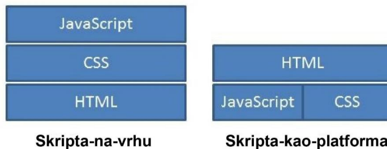
Slika 26. Skripta-na-vrhu i Skripta-kao-plaftoma arhitekture programskog jezika JavaScript (Izvor: Ince, 2011)
