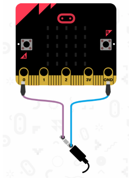
Slika 28. Prikaz pinova „0“ i GND sa spajanjem na kleme koje vode prema zvučniku
