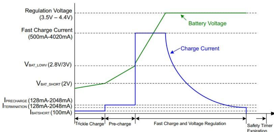
Slika 4: Graf napona i struje kroz četiri režima punjenja (Texas Instrument (2012.), I2C Controlled Single Cell USB/Adaptor Charger BQ24195 Datasheet , str.18)
