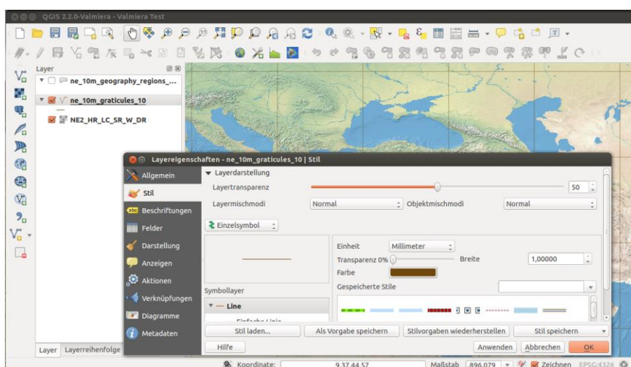
Slika 35 QGIS aplikacija
