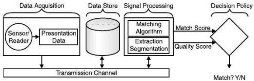
Slika 8.1.: Dijagram komponenata i toka biometrijskog sustava 12
