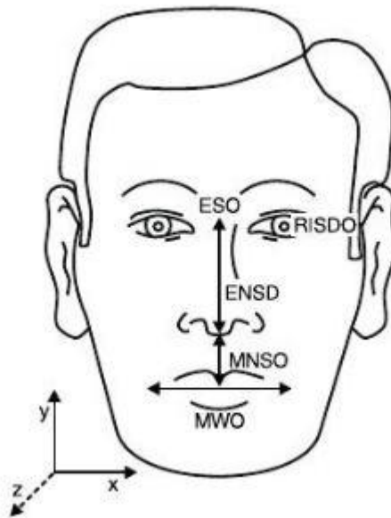
Slika 9.3.1.: Facial recognition
