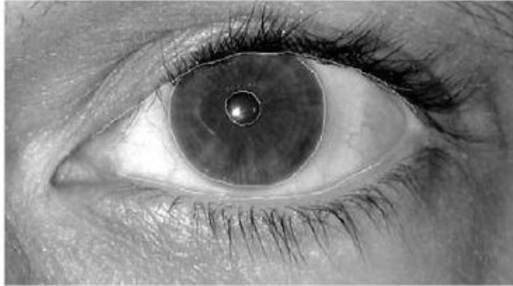
Slika 9.5.1.:Prepoznavanje šarenice
