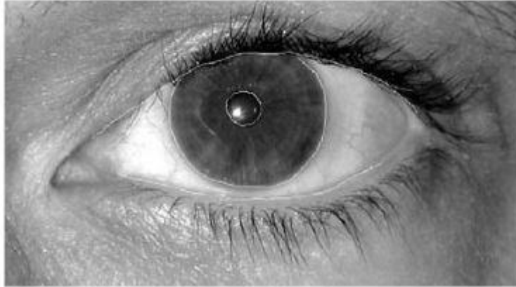
Slika 9.5.1.:Prepoznavanje šarenice
