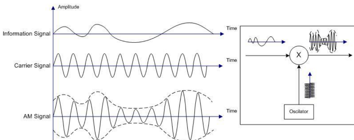
Slika 2. 4. Amplitudna modulacija
