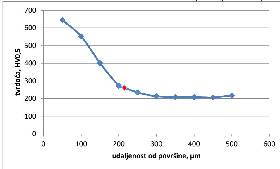
Slika 30. Ovisnost tvrdoće udaljenosti od površine za uzorak 1
