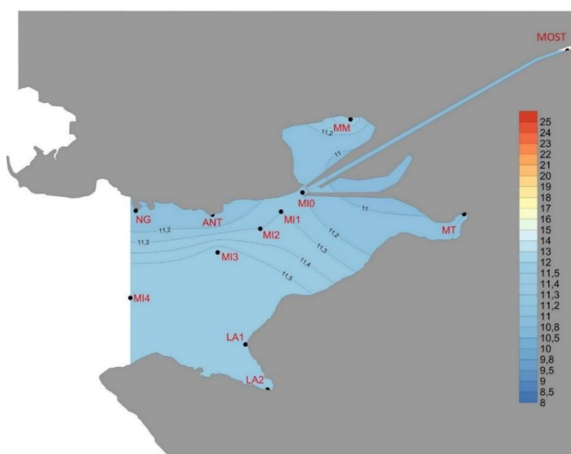
Slika 5. Raspodjela temperature ( T/^{\circ}\text{C} ) u površinskom sloju u veljači 2016.
