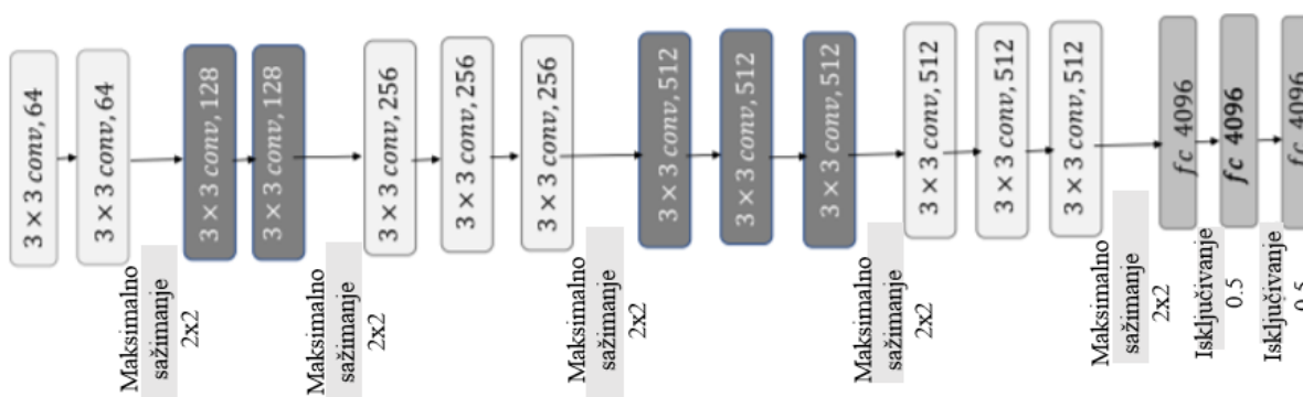
Slika 38. RGGF arhitektura
