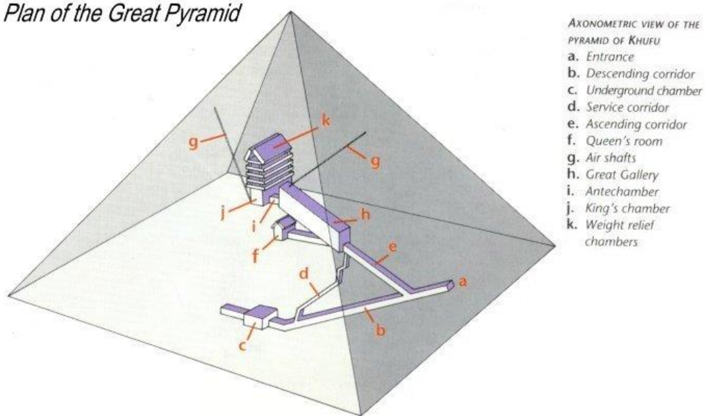
Slika 4. Unutrašnja struktura piramide
