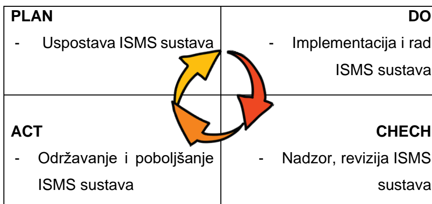
Slika 4: PDCA model
